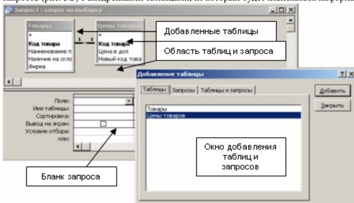
Рис. 5.3. Окно конструктора запросов Запрос на выборку и окно Добавление таблицы
