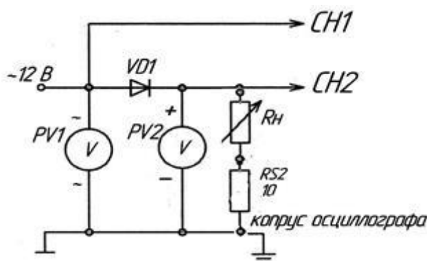
Рис.1. Схема для исследования однополупериодного выпрямителя на одном диоде.
