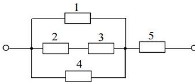
Рис. 1 Схема расчета надежности устройства
