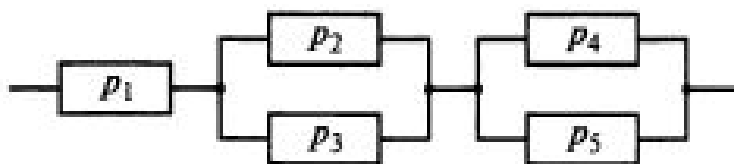
Рис. 1 Схема расчета надежности устройства
