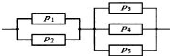
Рис. 1 Схема расчета надежности устройства
