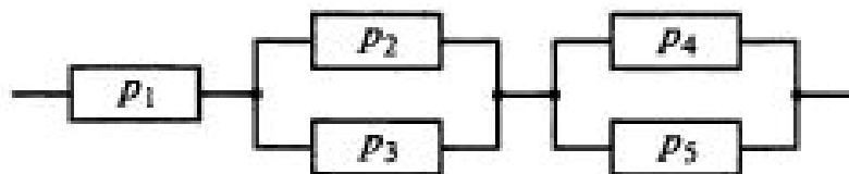
Рис. 1 Схема расчета надежности устройства
