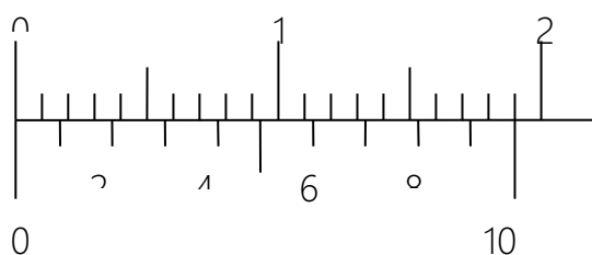
Рис. 1. Нониус с отсчётом до 0,1 мм
