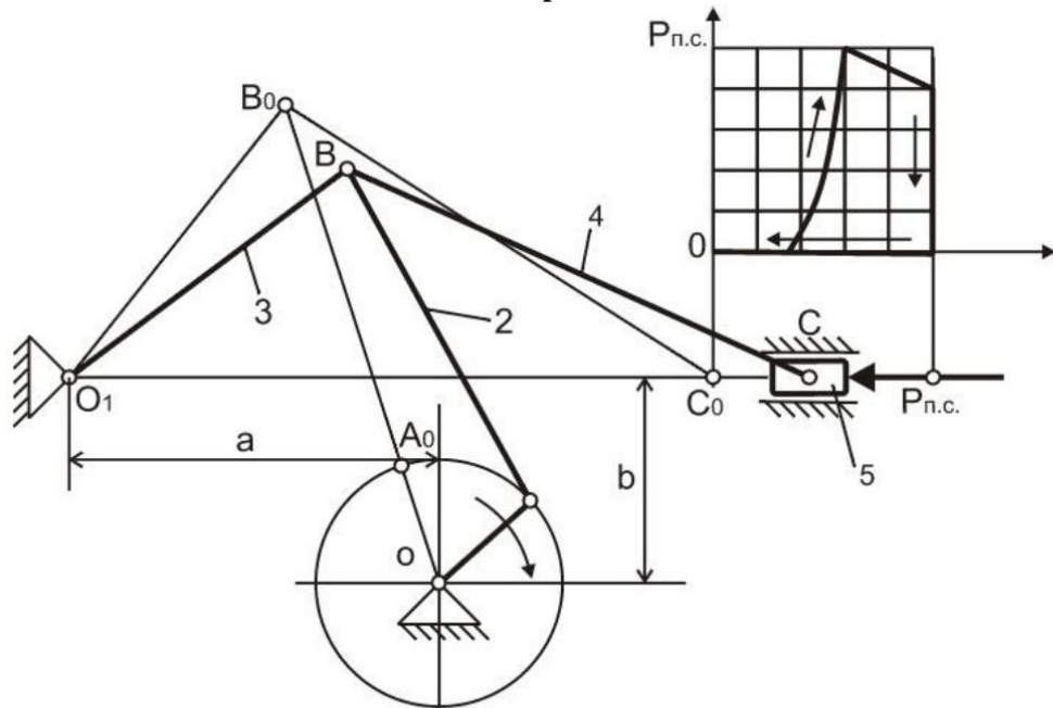
Механизм прессования
